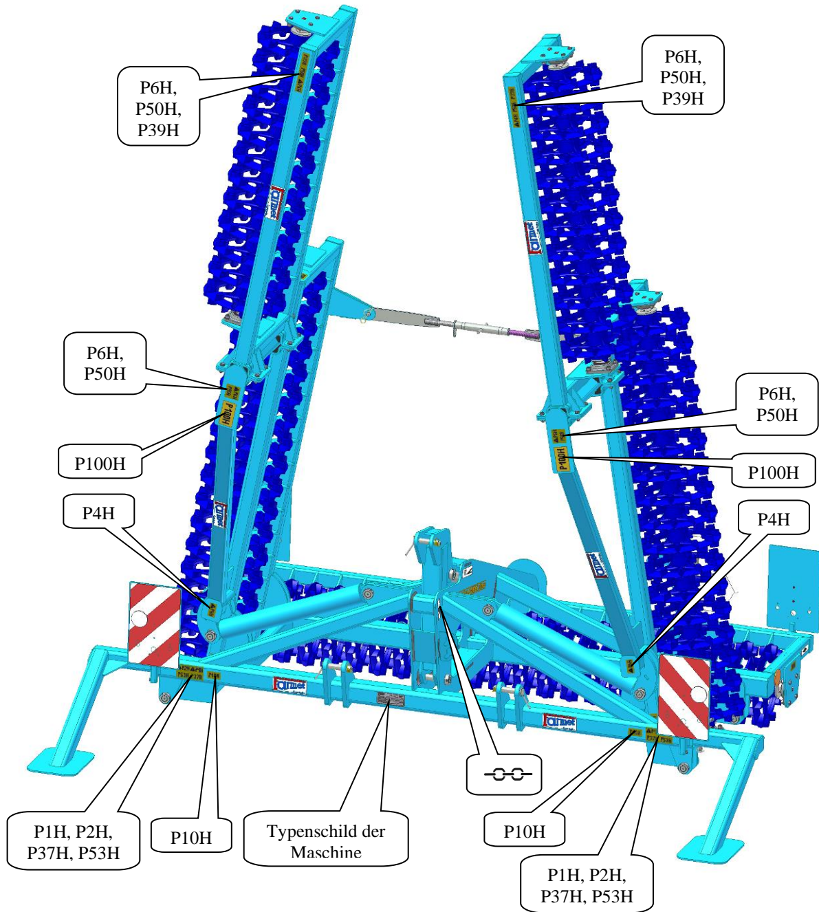
Abb.1-Anordnung der Sicherheitsschilder an der Maschine
