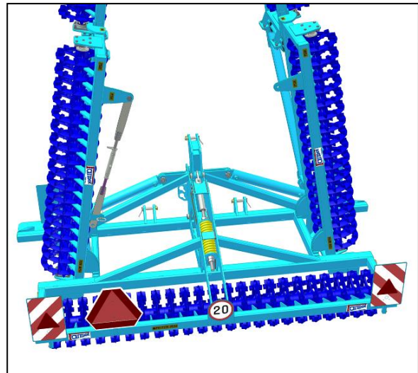
Abb. 6: Schwenkbereich der Maschine - nicht in den schraffierten Bereich eintreten
