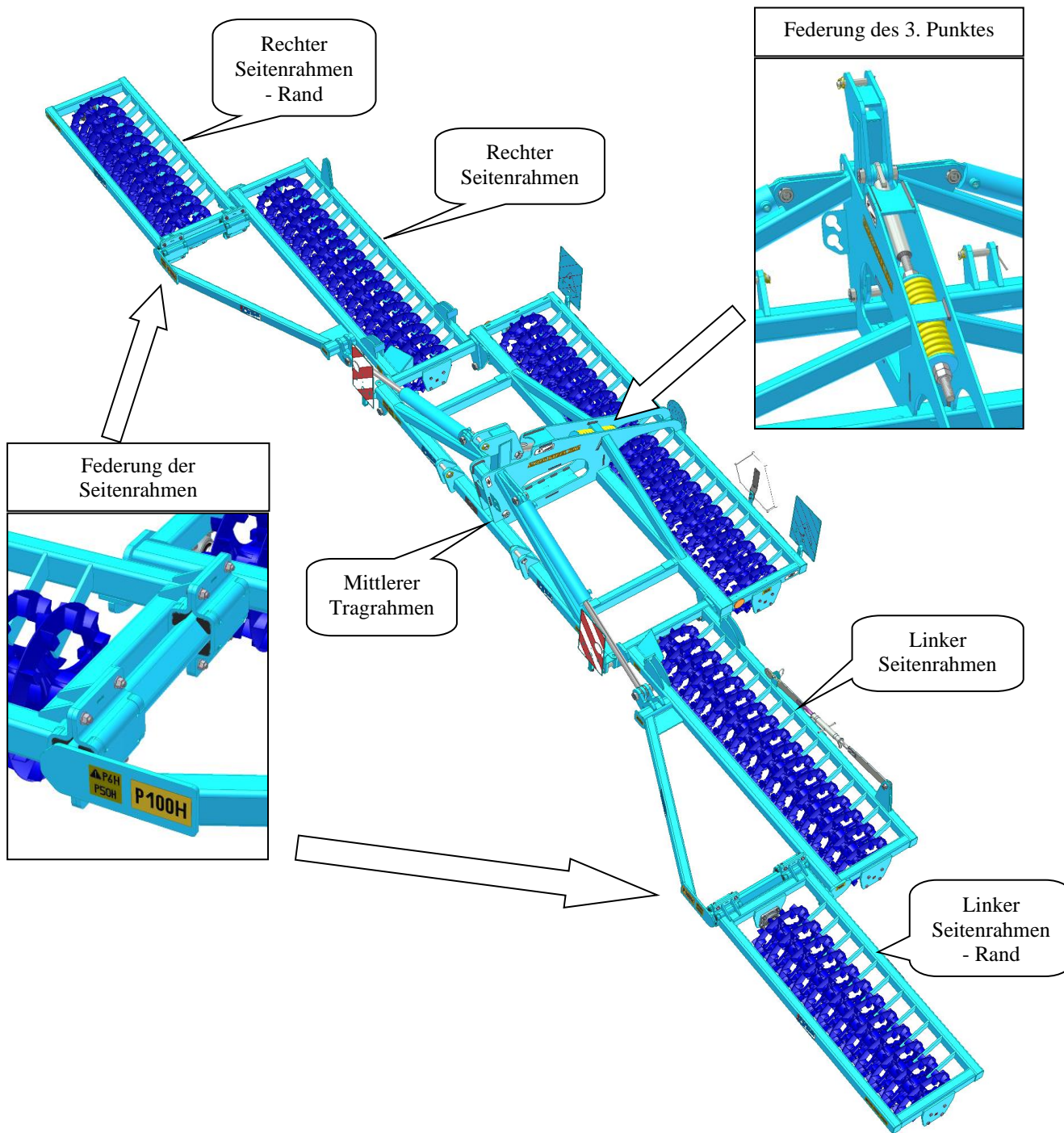
Abb. 3: Beschreibung der Maschine - aufgeklappt
